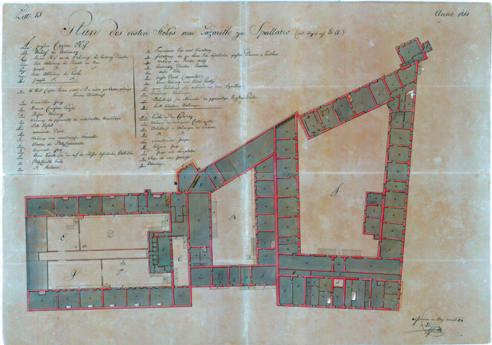
27. Walter Raughmann, Nacr prvog kata Generalata, carinarnice, priorata i prvog dvorišta karantene, 1814.
