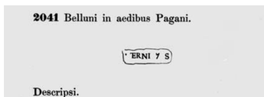
Fig. 1. La scheda di Theodor Mommsen (da CIL V 2041)
