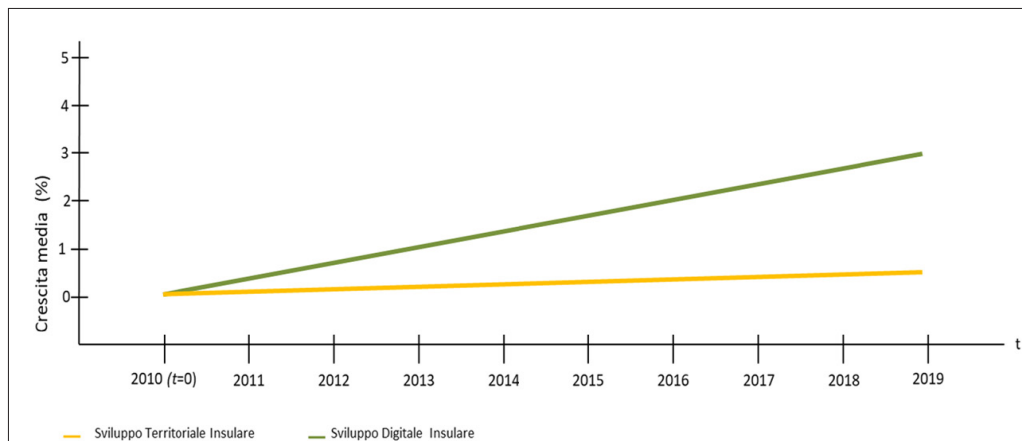
Fig. 1. Rappresentazione grafica dei risultati della ricerca. Comparazione tra Indicatore di Sviluppo Territoriale Insulare ( I_{STI} ) e Indicatore di Sviluppo Digitale Insulare ( I_{SDI} ).
