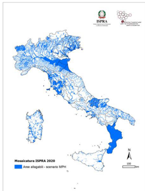
Fig. 1. Aree a pericolosità idraulica media P2 (D.Lgs. 49/2010); Fonte: Rapporto ISPRA, 356/2021.
