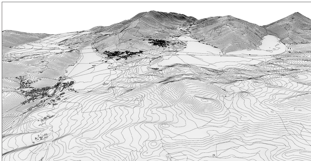
Fig. 2. Modello tridimensionale algoritmico dell'Altopiano delle Cinquemiglia (AQ).
