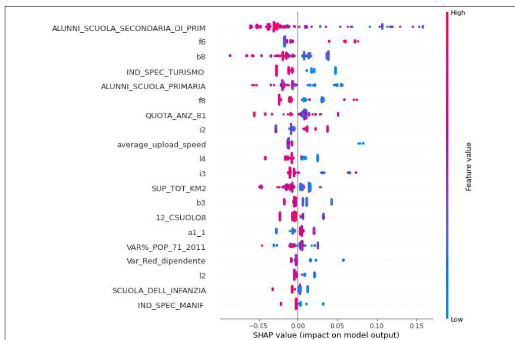
Fig. 2. Summary plot dei valori di Shapley per la descrizione delle aree marginali. Sull'asse delle ordinate sono presentate le variabili in ordine di importanza crescente mentre sull'asse delle ascisse è indicato l'impatto delle variabili sia in termini positivi che negativi sulle scelte del modello. Ciascun punto del grafico è un comune il cui valore alto o basso della variabile visualizzato è indicato dalla scala di colori.
