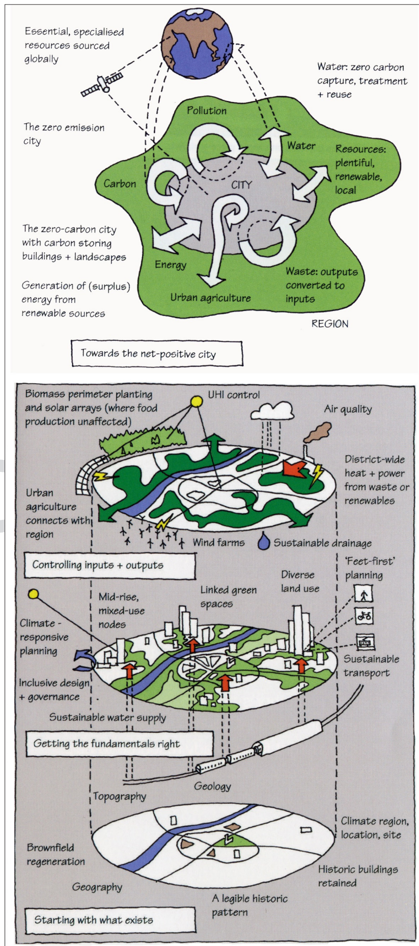
Fig. 2. Regole strategiche per città sostenibili. Verso le città net-positive. Fonte: H. Heywood (2015), 101 Rules of thumbs. For sustainable buildings and cities, RIBA Publishing, London.
